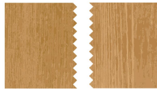
Zinkenverleimte Plattenverbindung garantiert hohe Festigkeit und maximale Verbindungssteifigkeit
