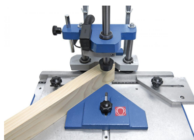
Max. Durchgangshöhe von 100 mm, max. Frästiefe 50 mm
