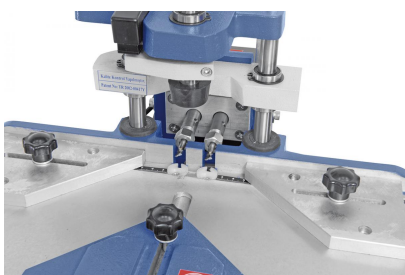
Gleichzeitige Herstellung von zwei Keilnuten mit fixem Spindelabstand von 28 mm
