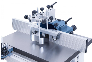
Die Fräuserschutzhaube ist mit eloxierten Aluminium-Anschlagsschienen ausgestattet.
