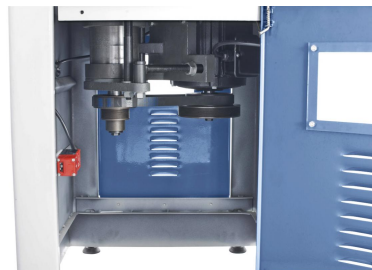
Schneller und einfacher Drehzahlwechsel mittels Keilriemen.
