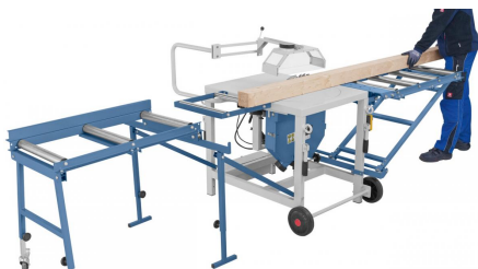
Paralleler Auftrennschnitt
