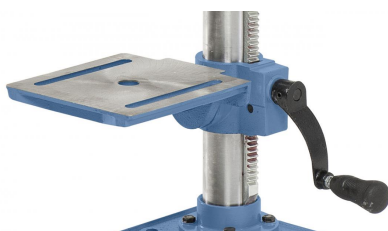
Der Bohrtisch ist von -45^\circ bis +45^\circ schwenkbar und 360^\circ um die Säule drehbar.
