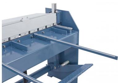
Problemloses Einrichten des Werkstückes durch Auflagearme mit Skalen.
