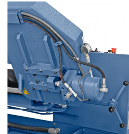
Optional mit hydraulischer Sägebandspannung lieferbar
