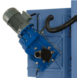
Leistungsstarker Antriebsmotor mit schräg verzahntem Getriebe, Antriebsleistung 4,0 kW
