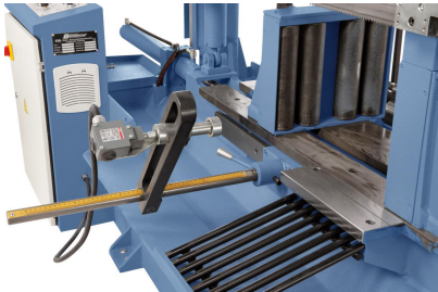
Manuelle Voreinstellung der Materiallänge mittels Mikroschalter, Eingabe und Kontrolle der Stückzahl am Bedienpult
