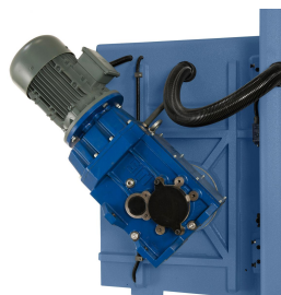
Leistungsstarker Antriebsmotor mit schräg verzahntem Getriebe, Antriebsleistung 3,0 kW
