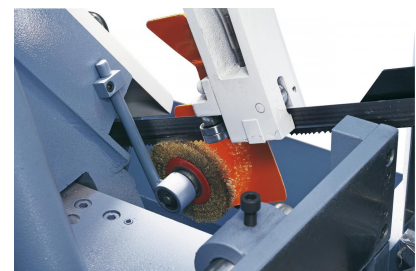
Kugelgelagerte Sägebandführung und Spänebürste für optimale Schnittergebnisse.
