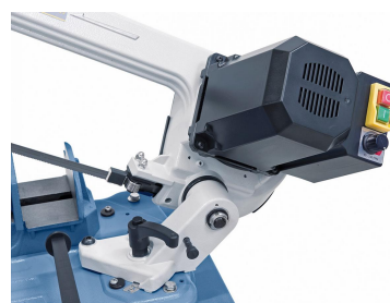
Leistungsstarker Antriebsmotor mit elektronischem Drehzahlregler.
