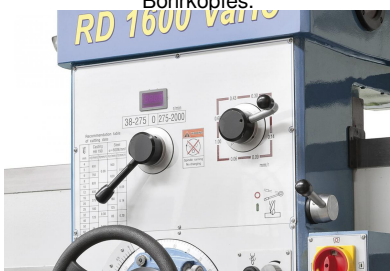
Die Einstellung der gewünschten Drehzahl bzw. des Vorschubs erfolgt an der Vorderseite
