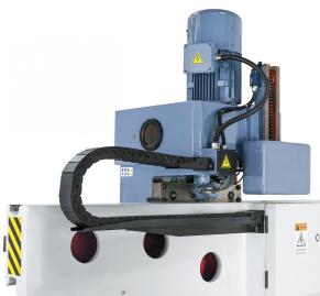
Gegengewicht für die Pinole und Energieführungskette an der Rückseite des Bohrkopfes.
