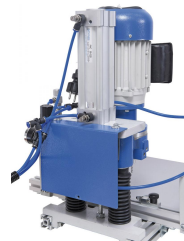
Wartungsfreier Aluminium-Vorschubzylinder
