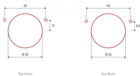
Scharnertypen
