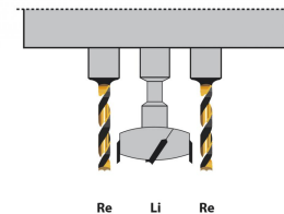
Der zentrale Beschlagbohrer ist linksdrehend, die beiden äußeren Bohrer rechtsdrehend
