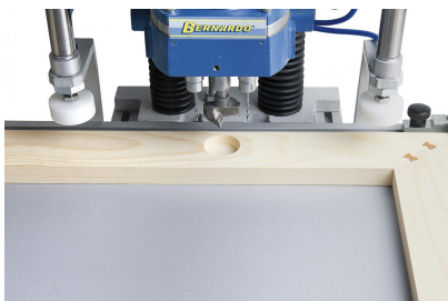
Inklusive Klappanschläge, ideal für Serienarbeiten
