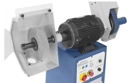
Verstellbare Schutzhaube mit Schutzvorrichtung und Absauganschluss
