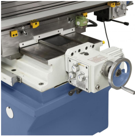
Robuster Tischvorschub in y-Achse mit Eilgangfunktion.
