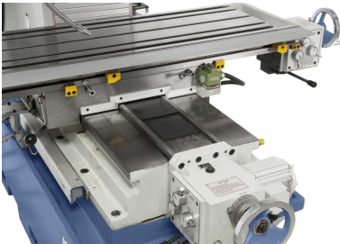
Leichte und gleichmäßige Tischverstellung durch stabile Flachführung in der y-Achse.
