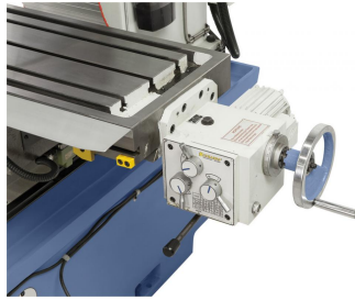
Die Tischverstellung in x-Achse erfolgt über 8 frei wählbare Vorschübe (24 - 720 mm/min).
