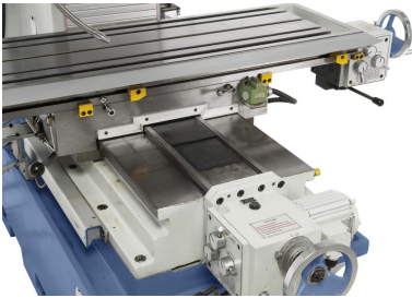
Leichte und gleichmäßige Tischverstellung durch stabile Flachführung in der y-Achse.
