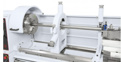
Serienmäßig mit feststehender Lünette zum Einspannen von langen Werkstücken.
