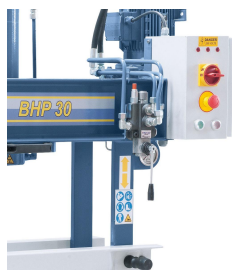
Ein feinfühliges Zustellen und Stoppen des Kolbens wird mittels Spezialhebel gewährleistet.
