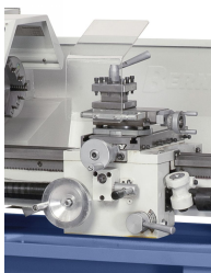
Ergonomisch angebrachte Schaltehebel zur Einstellung des Längs- und Quervorschubes.
