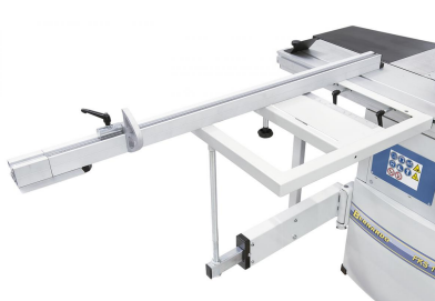
Der stufenlos schwenkbare (2x 45°) Teleskopanschlag kann wahlweise vorne oder hinten am Besäumrahmen montiert werden.
