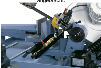
Für feinfühliges Absenken des Sägebügels serienmäßig mit Hydraulikzylinder
