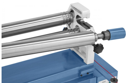
Nach vorne ausschwenkbare Oberwalze zur leichten Entnahme des fertigen Werkstückes.
