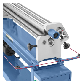
Einfache Zustellung der Unter- und Hinterwalze mittels Handgriffe.
