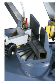
Der Sägebügel kann für Gehrungsschnitte von 90° bis 60° verstellt werden.
