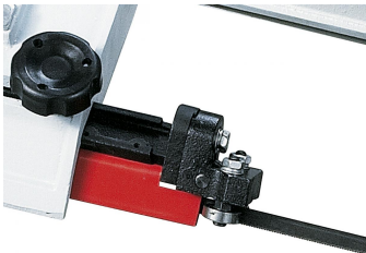
Kugelgelagerte Sägebandführung, einstellbar auf die jeweilige Werkstückbreite.
