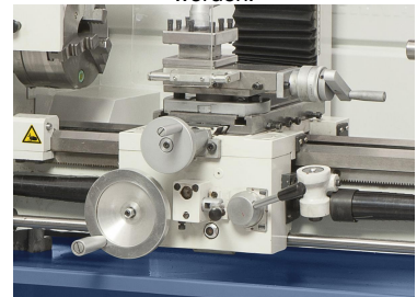
Schlitten inkl. Handräder mit Feinskalierung. Zusätzlich ist dieses Modell mit einem automatischem Quervorschub ausgestattet.
