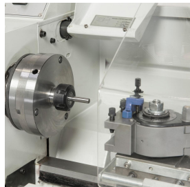
Optional lieferbar: Schnellwechselstahlhalter System Multifix und Spannzangenfutter ER 25
