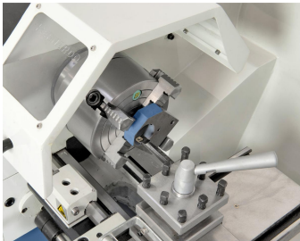
Planscheibe 160 mm (Option) ideal zum Aufspannen von asymmetrischen Werkstücken.
