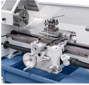
Ergonomisch angebrachte Schalthebel zur Einstellung des Längs- und Quervorschubes.
