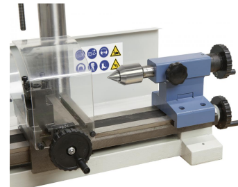
Reitstock mit Tiefenskala und optional lieferbarem Rollkörper MK 1
