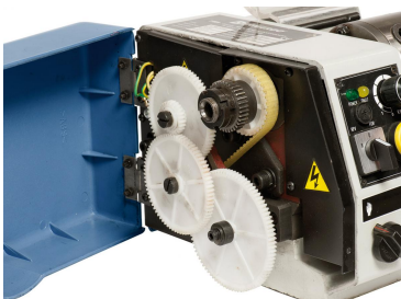
Optional mit Wechselräder zum Gewindeschneiden (Steigung von 0,5 - 1,25 mm)
