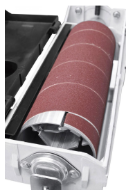
Schnellspannsystem zum Befestigen des Schleifbandes.
