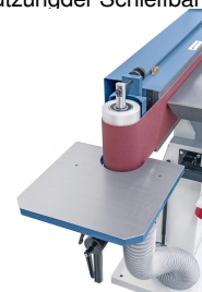
Rundschleiftisch mit Absauganschluss ideal zum Schleifen von Radien und Konturen.
