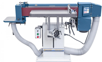
Höhenverstellbarer Arbeitstisch zur optimalen Ausnutzung der Schleifbandbreite.
