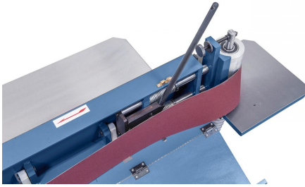
Bedienerfreundliches Wechseln des Schleifbandes durch Schnellspanneinrichtung.
