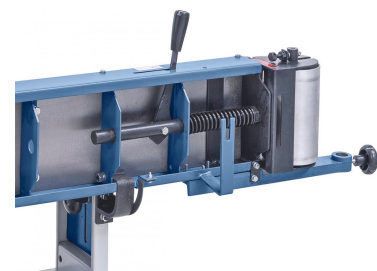
Gefederte Bandspannung, dadurch automatischer Ausgleich von Bandlängendifferenzen.
