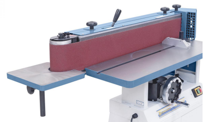
Der höhenverstellbare Zusatztisch ermöglicht das Schleifen von Konturen an der Umlenkrolle
