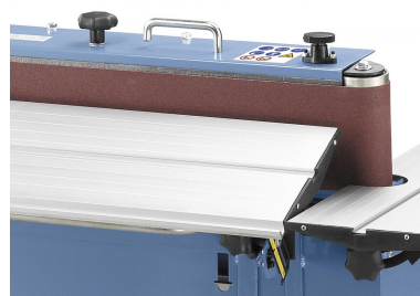
Der Arbeitstisch ist von 0° bis 45° schwenkbar
