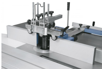
Massive Fräuserschutzhaube mit feineinstellbaren Anschlagsschienen.
