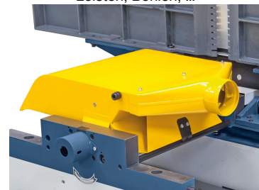
Integrierte umklappbare Spanauswurfhaube -
