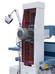
Geschliffene Flachführung für exaktes Zustellen des Schleifkopfes.
