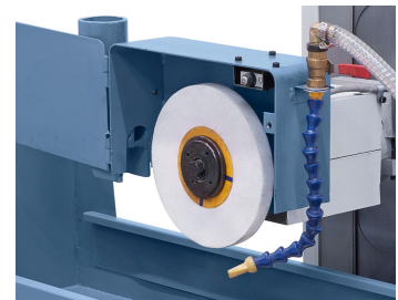
Vibrationsarmer Lauf und hohe Genauigkeit der Schleifspindel durch die vorgespannten Speziallager.
