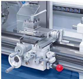
Leichtgängiger Schlitten mit Obersupport und Vierfachstahlhalter, Handräder mit einstellbarer metrischer Feinskalierung
