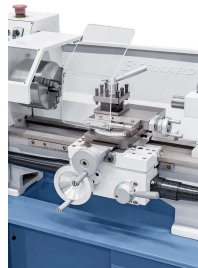
Leichtgängiger und präziser Schlitten mit Obersupport, lange Lebensdauer durch spielfrei nachstellbare Keilleisten
