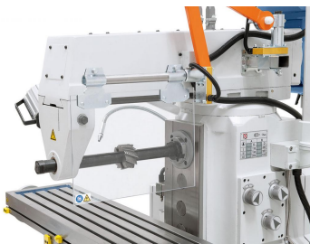
Zum Fräsen in horizontaler Position serienmäßig mit Gegenlager und langem Fräsdorn.
