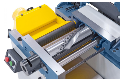
Das Hobelwerk besteht aus einer dynamisch ausgewuchteten Spiralmesser-Hobelwelle, einer Ein- und Auszugswalze, sowie massiven Rückschlagsicherungen.
