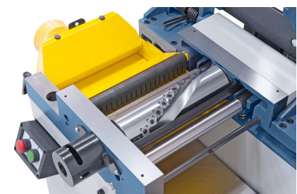
Das Hobelwerk besteht aus einer dynamisch ausgewuchteten Spiralmesser-Hobelwelle, einer Ein- und Auszugswalze, sowie massiven Rückschlagsicherungen.
