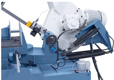
Serienmäßig mit Hydraulikzylinder zum feinfühligem Absenken des Sägebügels.
