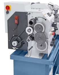
Zum Bearbeiten von großen Wellendurchmessern serienmäßig mit einer 38 mm Spindelbohrung ausgestattet.
