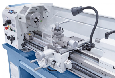
Ergonomisch angebrachte Schalthebel zur Einstellung des Längs- und Quervorschubes.
