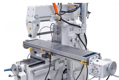
Serienmäßig mit Gegenlager und langem Fräsdorn für horizontale Fräsarbeiten.
