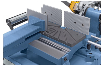
Schraubstock mit Schnellarretierung zum Doppelgehrungsschneiden verschiebbar
