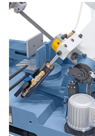
Hydraulikzylinder für stufenloses Absenken des Sägebügels.
