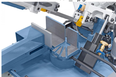
Schwenkbarer Sägebügel für Gehrungsschnitte bis 45°
