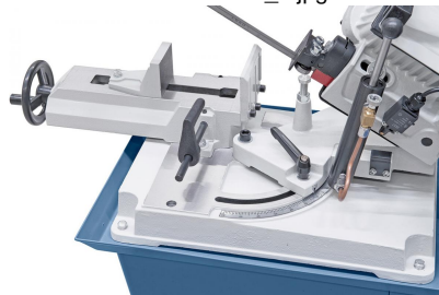
Schwenkbarer Sägebügel zum Gehrungsschneiden von +45° bis -60° verstellbar.
