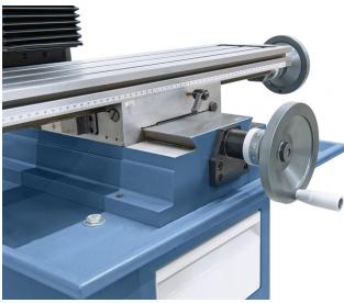
Schwalbenschwanzführung für x-, y- und z-Achse, nachstellbar über Keilleisten
