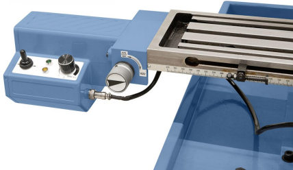
Für erhöhten Bedienkomfort optional mit stufenlos regelbarem Frästischvorschub FTV 9.
