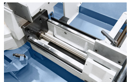
Präzisions-Linearführung mit Kugelumlaufspindel und leistungsstarkem Servo-Antrieb für höchste Positioniergenauigkeit des Werkstückes.
