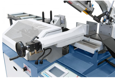
Hydraulischer Schraubstock zum Gehrungsschneiden verschiebbar.
