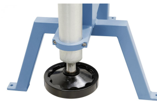
Einfaches Einstellen der unteren Formrolle mittels Fußrad.
