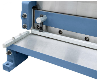
Automatisch wirkender Niederhalter zum Fixieren des Bleches.
