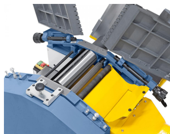
Die dynamisch ausgewuchtete 3-Messerwelle garantiert durch den vibrationsfreien und ruhigen Lauf beste Hobelergebnisse
