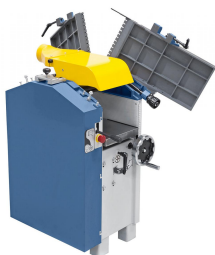
Die hochklappbaren Abrichttische ermöglichen beim Dickenhobeln ein optimales und sicheres Arbeiten, auch bei kurzen Werkstücken
