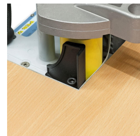
Serienmäßig mit Führungsplatte zum Anbringen des Kanten-materials in Ecken.
