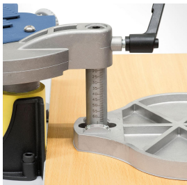
Höhenverstellbare Führungsplatte mit Skala zum Einstellen des zu bearbeitenden Werkstücks
