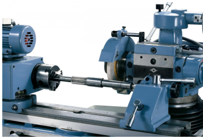
Außenrundsleifen
