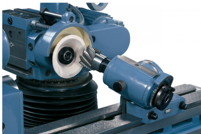
Werkzeugschleifen
