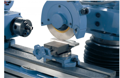
Flachsleifen
